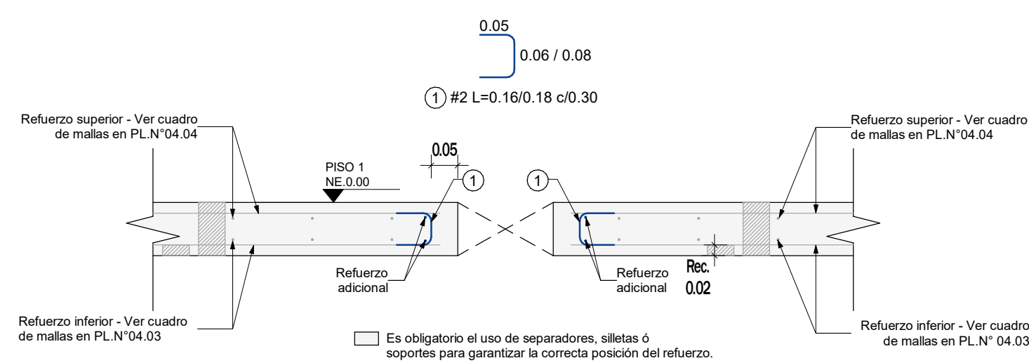
DETALLE TÍPICO - UBICACIÓN REFUERZO ADICIONAL
