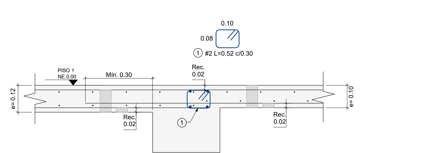
DETALLE TÍPICO - CAMBIO DE SECCIÓN
