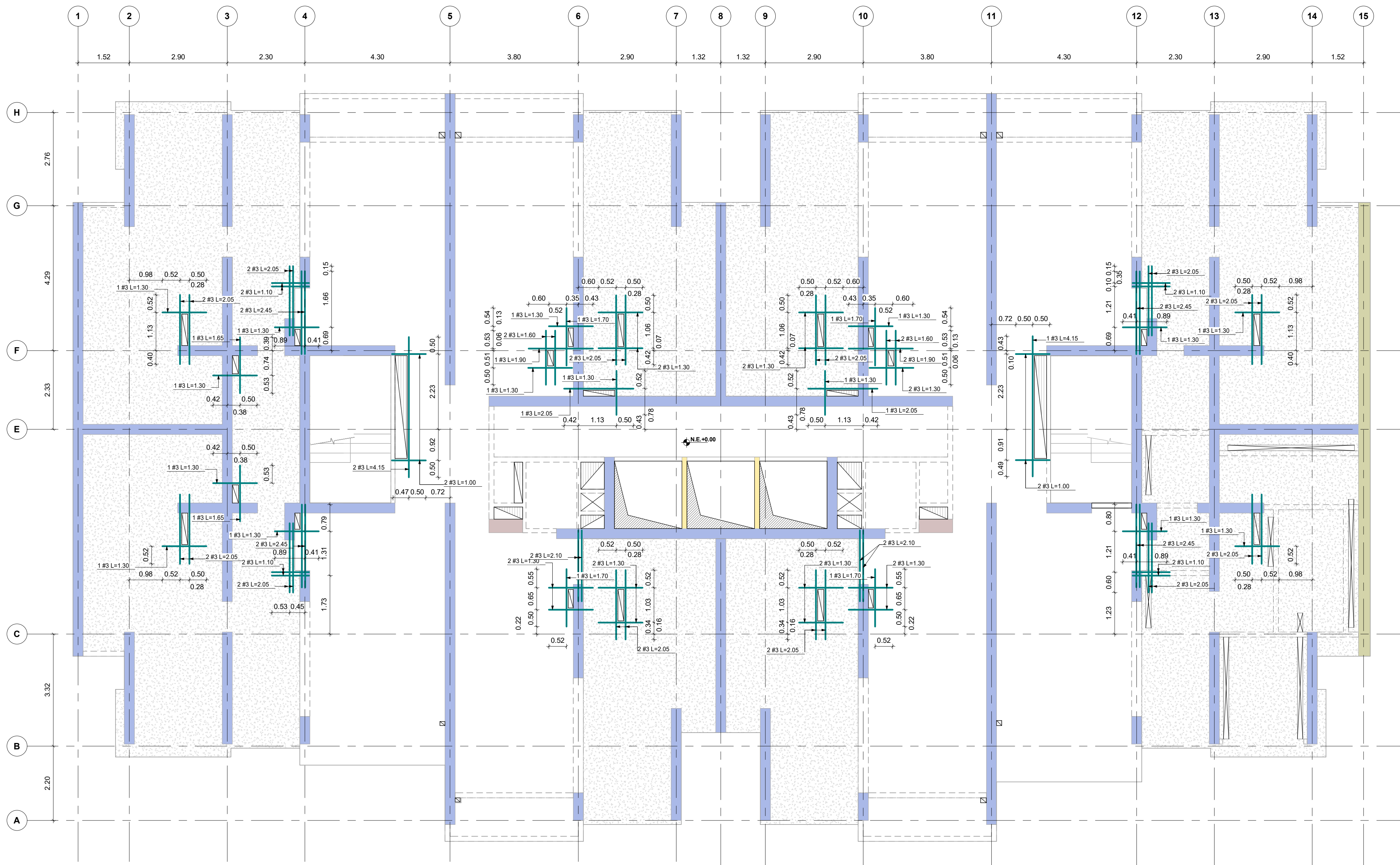
PLANTA DE REFUERZO ADICIONAL (INFERIOR Y SUPERIOR) PISO 1 N.E. 0.00
