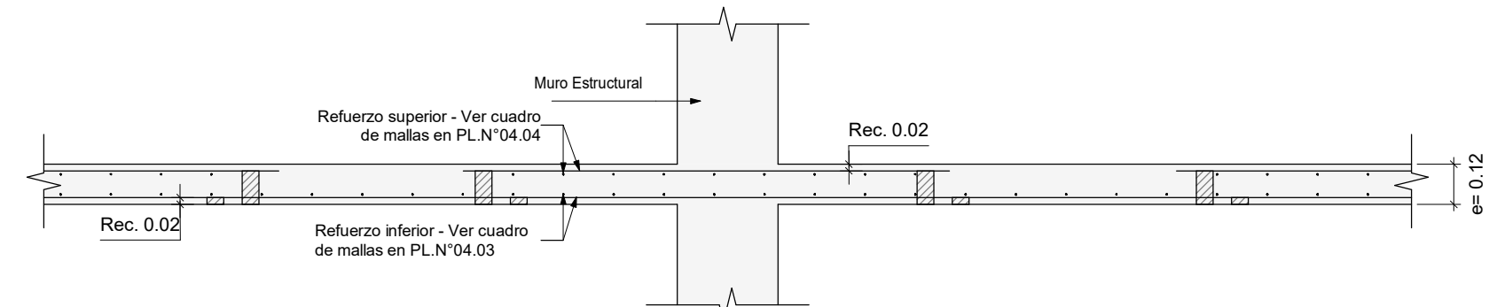
CORTE TÍPICO PLACA AÉREA e=0.12
