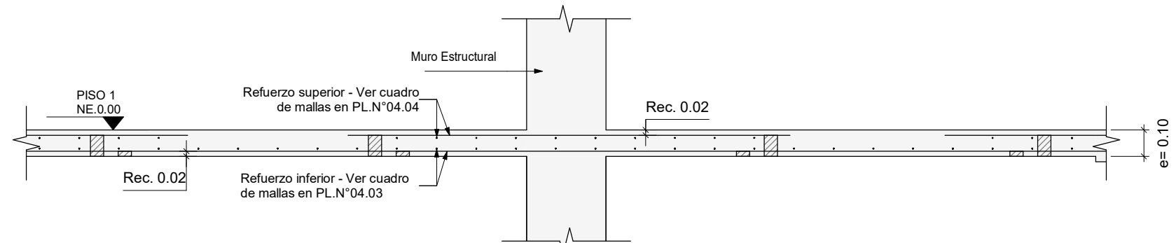
CORTE TÍPICO PLACA AÉREA e=0.10
